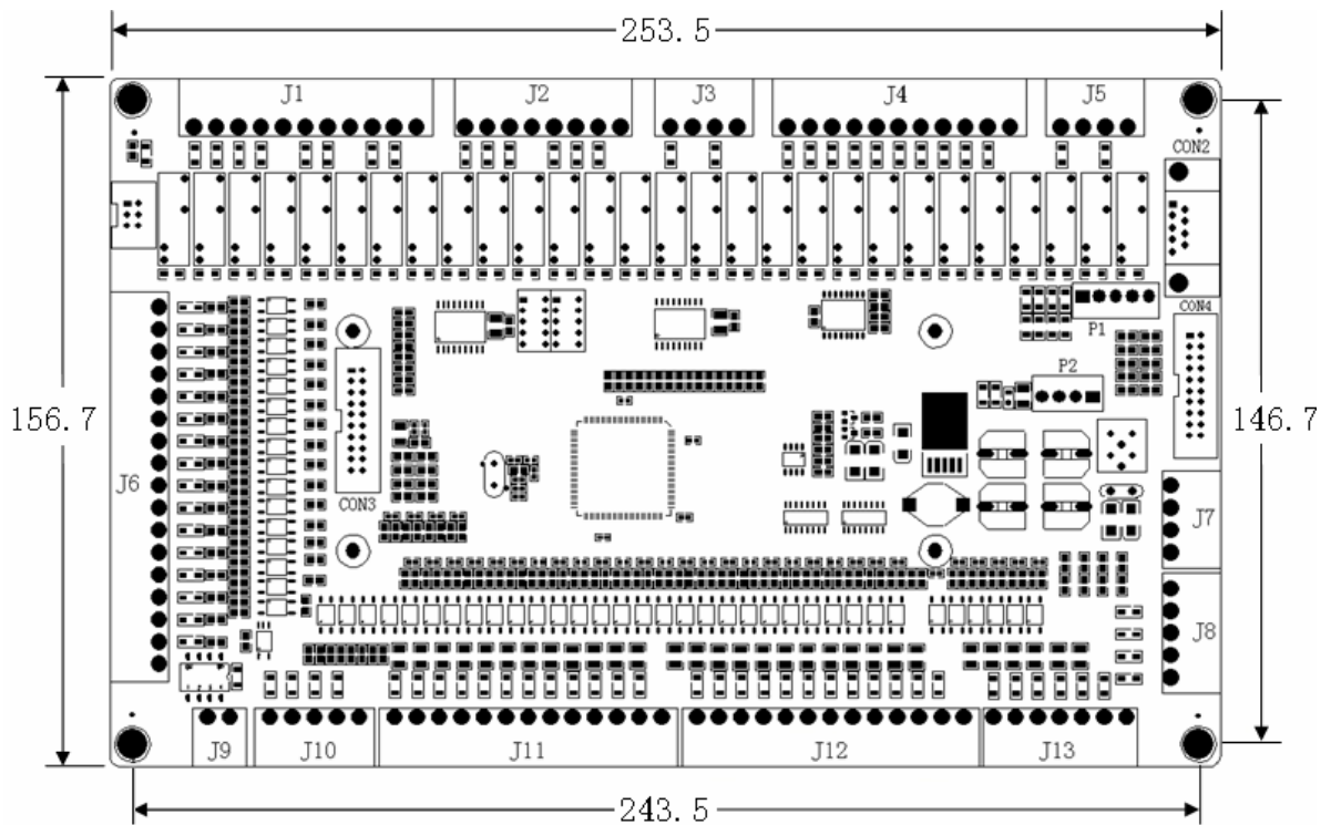
ME-LIFT-P 外观显示图
